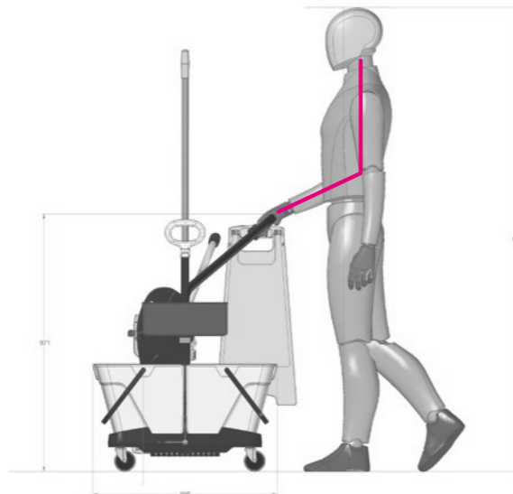
50. Perzentil männlich | Neigung des Unterarms beim Schieben.
