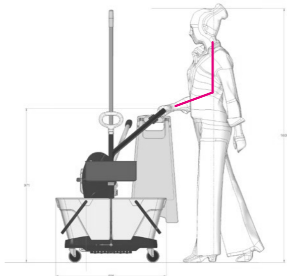
50. Perzentil weiblich | Neigung des Unterarms beim Schieben.
